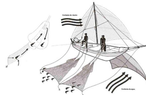
Esquema de las atarrayas "Suripera", demostrando su principio operativo
